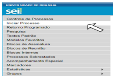
Figura 1: Iniciar Processo
